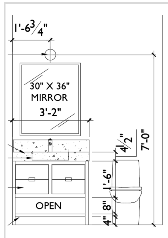
ELEVATION
